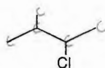
2-chloro-3-methylbutane
